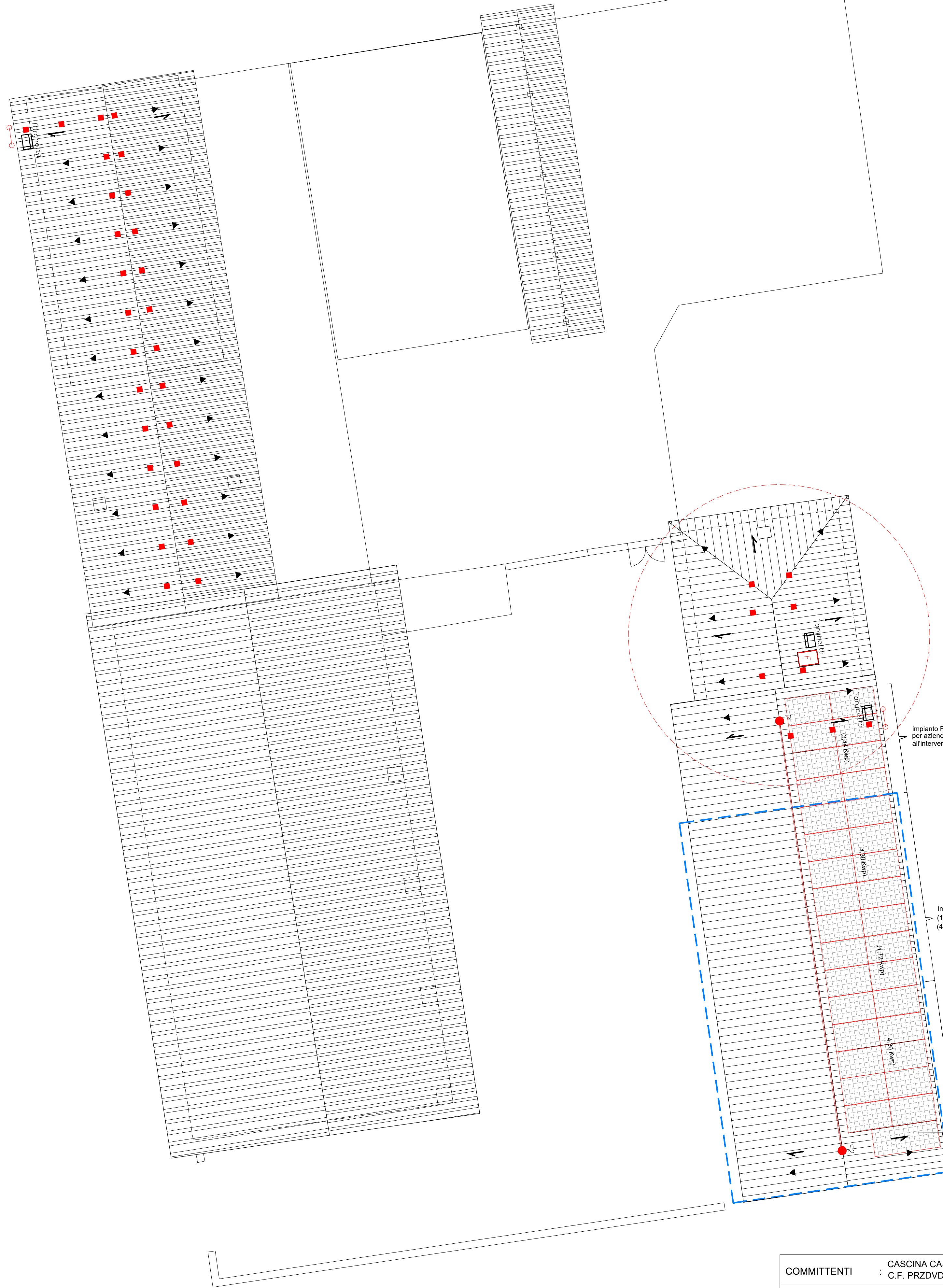
PROGETTO PIANTA COPERTURE - SCHEMA FOTOVOLTAICO E SOLARE TERMICO SCHEMA LINEA VITA scala 1 : 100
